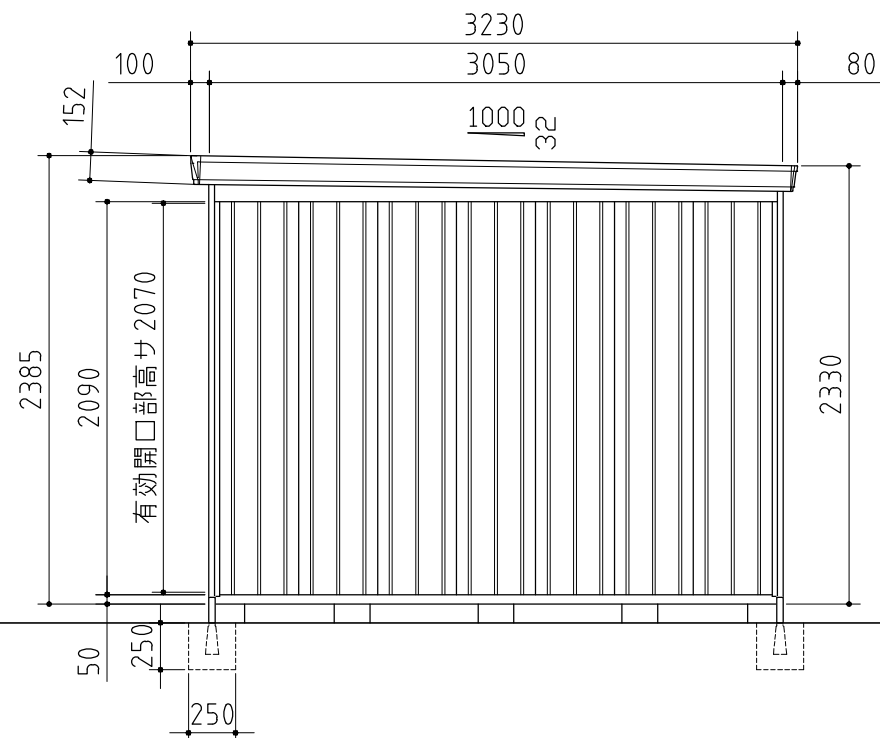
側面図
